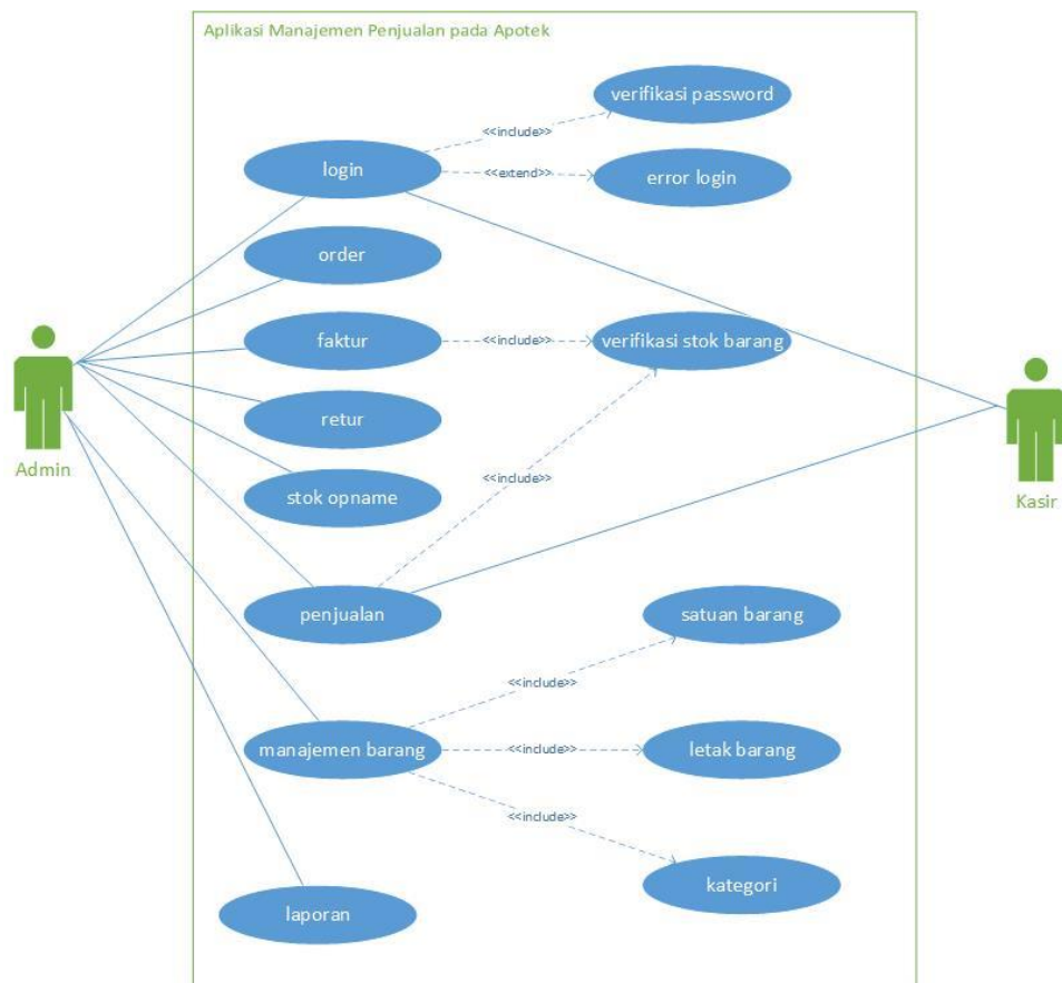
Gambar 4 Use Case Diagram Aplikasi
