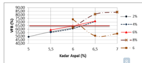
Gambar 6 Kurva Hubungan VFB dengan Kadar Aspal
