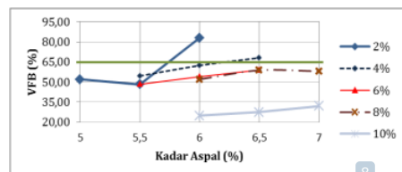
Gambar 12 Kurva Hubungan VFB dengan Kadar Aspal
