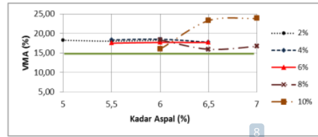
Gambar 5 Kurva Hubungan VMA dengan Kadar Aspal
