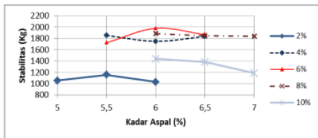
Gambar 7 Kurva Hubungan Stabilitas dengan Kadar Aspal
