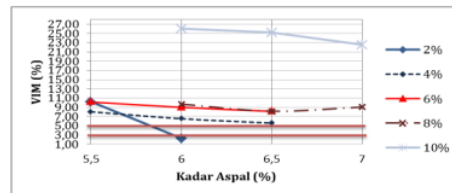
Gambar 10 Kurva Hubungan VIM dengan Kadar Aspal
