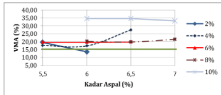
Gambar 11 Kurva Hubungan VMA dengan Kadar Aspal
