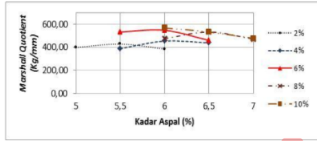
Gambar 3 Kurva Hubungan Marshall Quotient dengan Kadar Aspal
