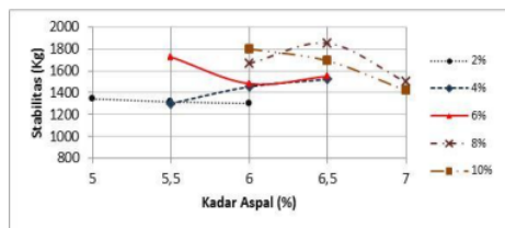
Gambar 1 Kurva Hubungan Stabilitas dengan Kadar Aspal
