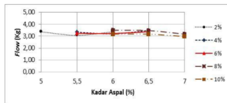
Gambar 2 Kurva Hubungan Flow dengan Kadar Aspal
