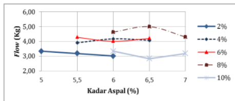
Gambar 8 Kurva Hubungan Flow dengan Kadar Aspal
