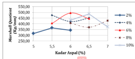
Gambar 9 Kurva Hubungan Marshall Quotient dengan Kadar Aspal
