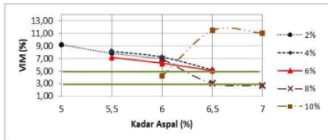
Gambar 4 Kurva Hubungan VIM dengan Kadar Aspal
